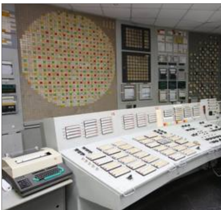
Dans la salle de contrôle du bloc n° 1, arrêté depuis 1996, la représentation du réacteur de type RBMK reproduite au mur.
